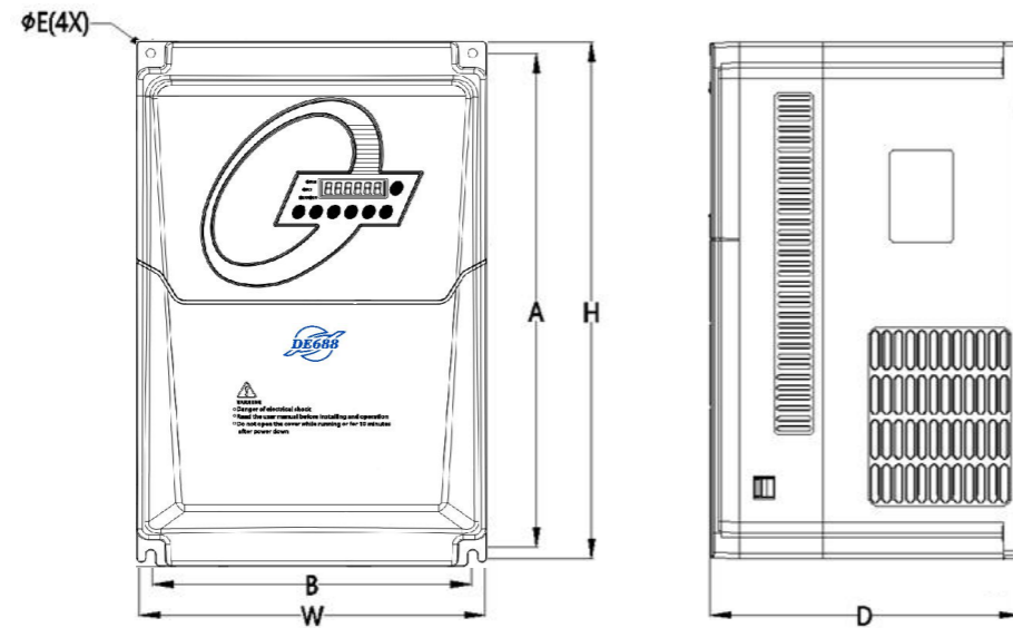
380V 11~37 kW 安装尺寸图 220V 11~22kW 安装尺寸图
