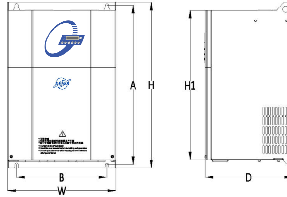
380V 45~90 kW 安装尺寸图 220V 30~55kW 安装尺寸图
